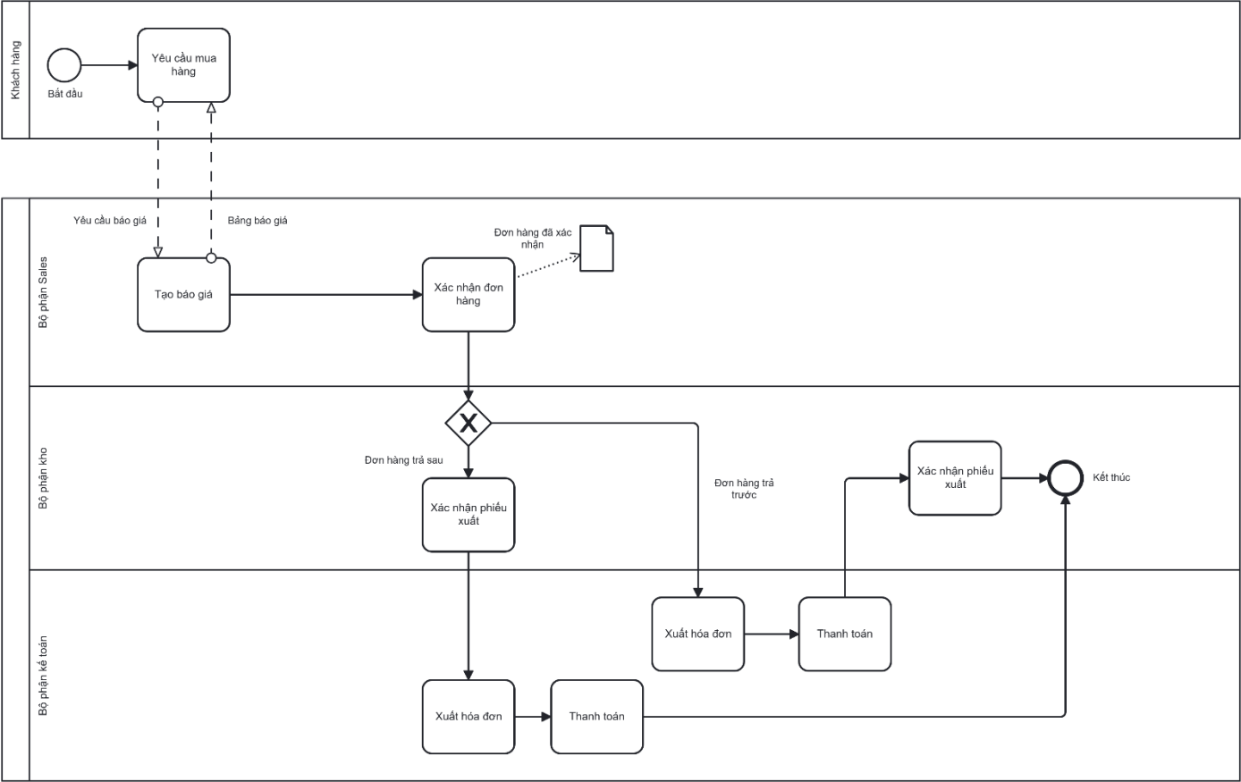
Hình 3.2 BPMN quy trình bán hàng
