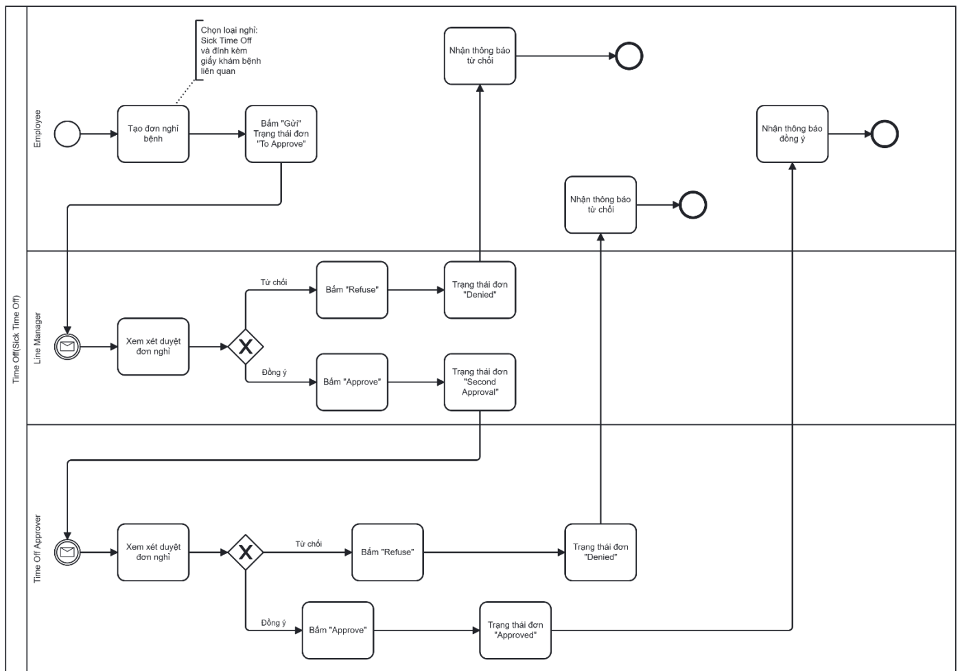
Hình 3.7 BPMN quy trình Nghỉ phép (Nghỉ ốm)
