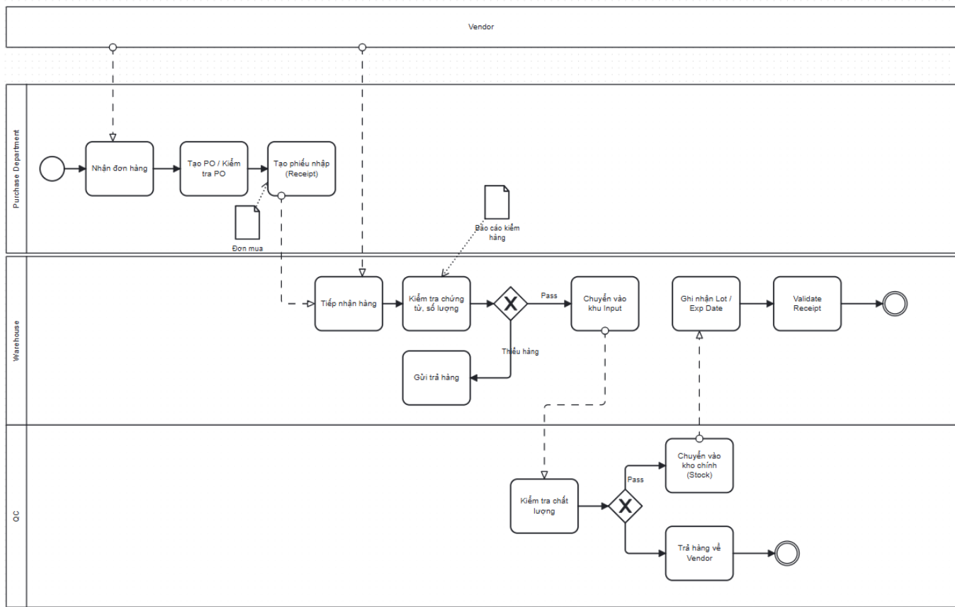
Hình 3.4 BPMN mô tả quy trình nhập kho
