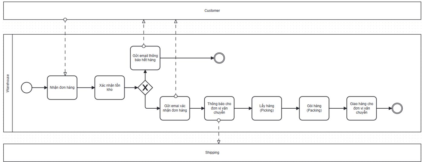
Hình 3.5 BPMN mô tả quy trình xuất kho
