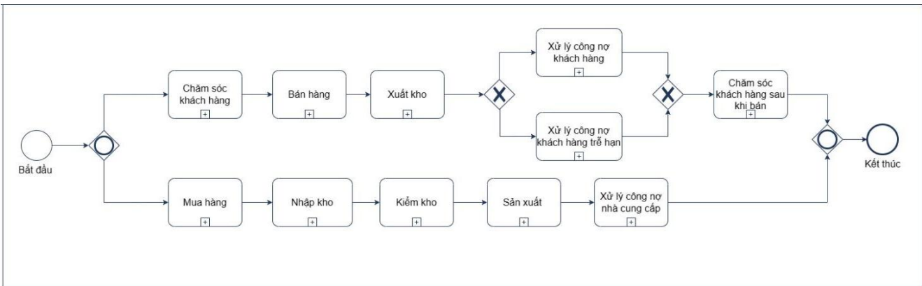
Hình 3.1 BPMN tổng quan quy trình
