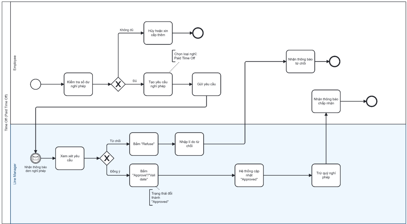
Hình 3.6 BPMN quy trình Nghỉ phép (Nghỉ phép có lương)
